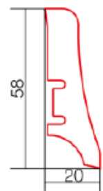
P 20 Profil
