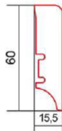
P6P Profil
